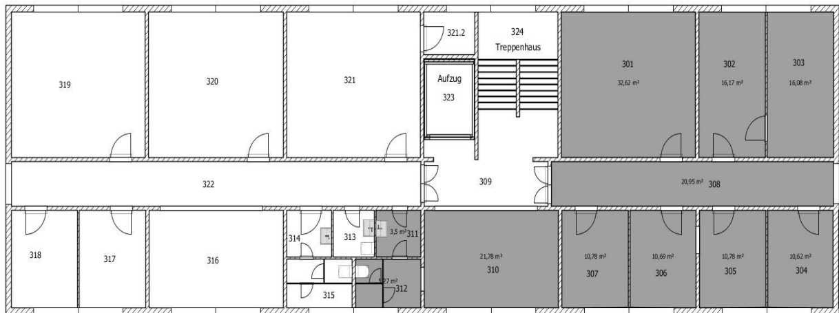
Grundriss 2.Obergeschoss Ätztehaus Fürstenberg
